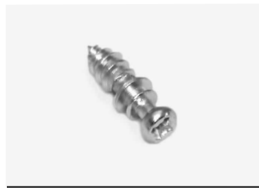
Vijak stezni fi 20 M6x12mm za ekscentar
